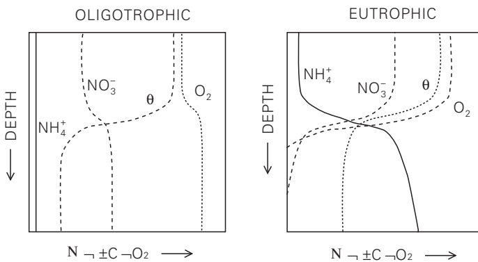
2. Fig. Oligotrofiko eta eutrofikoak diren laku estratifikatueta azal daitezkeen nitrato eta amonioaren soslai bertikal idealizatuak (Wetzel, 1975).
