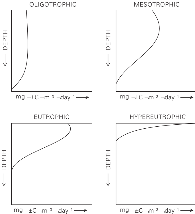
6. Fig. Eutrofia areagotzen ari den lakuetan azal daitezkeen ekoizpen fitoplanktonikoaren (ur-bolumen unitateko) soslai bertikal idealizatuak (Wetzel, 1975).
