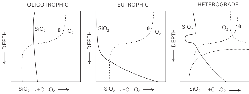
5. Fig. Oligotrofiko, eutrofiko eta banaketa heterogradokoak diren laku estratifikatuetan azal daitezkeen silizearen soslai bertikal idealizatuak (Wetzel, 1975).
