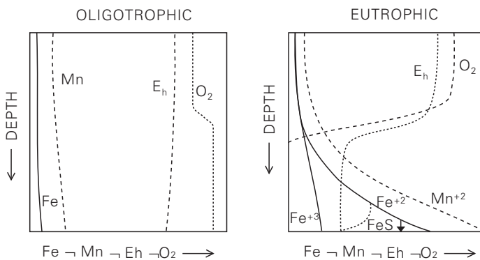
4. Fig. Oligotrofiko eta eutrofikoak diren laku estratifikatueta azal daitezkeen burdina, manganeso eta redox potentzialaren soslai bertikal idealizatuak (Wetzel, 1975).
