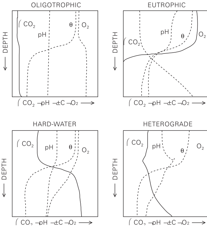
1. Fig. Oligotrofiko, eutrofiko, kalkareo eta banaketa heterogradokoak diren laku estratifikatueta azal daitezkeen oxigeno disolbatu, karbono inorganiko eta pH-aren soslai bertikal idealizatuak (Wetzel, 1975).
