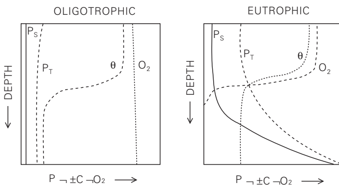
3. Fig. Oligotrofiko eta eutrofikoak diren laku estratifikatueta azal daitezkeen fosforo totala eta fosforo disolbagarriaren soslai bertikal idealizatuak (Wetzel, 1975).
